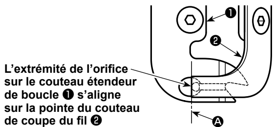
État d'alignement de la partie saillante du couteau étendeur de boucle et du couteau de coupe du fil
