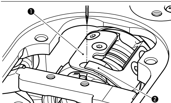
État d'alignement de la partie saillante du couteau étendeur de boucle et du couteau de coupe du fil
