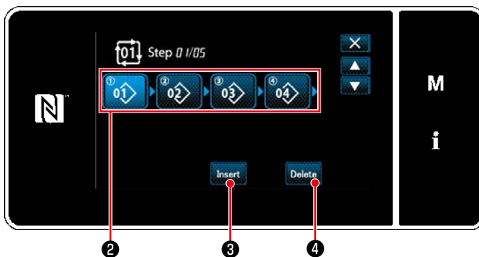
<Écran de modification des étapes de couture par cycles>
