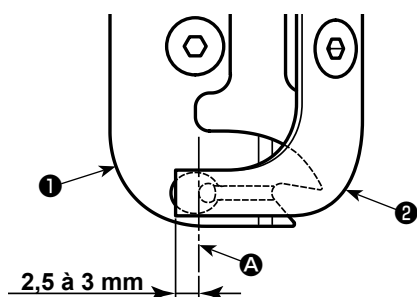
État de l'engagement du couteau
