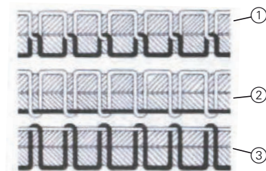
(1) - Tension du fil d'aiguille et du fil de crochet pareille
