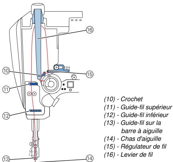
Fig. 8: Schéma d'enfilage - partie 2
