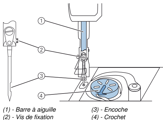
Fig. 3: Insérer et changer d'aiguille sur les machines à une aiguille
